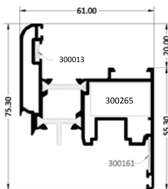
HOJA PUERTA CURVA CAN/16
