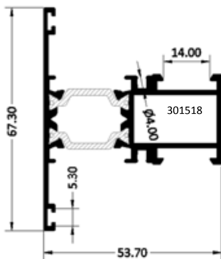
TRAVESAÑO VENTANA 67 MM CAN/16
