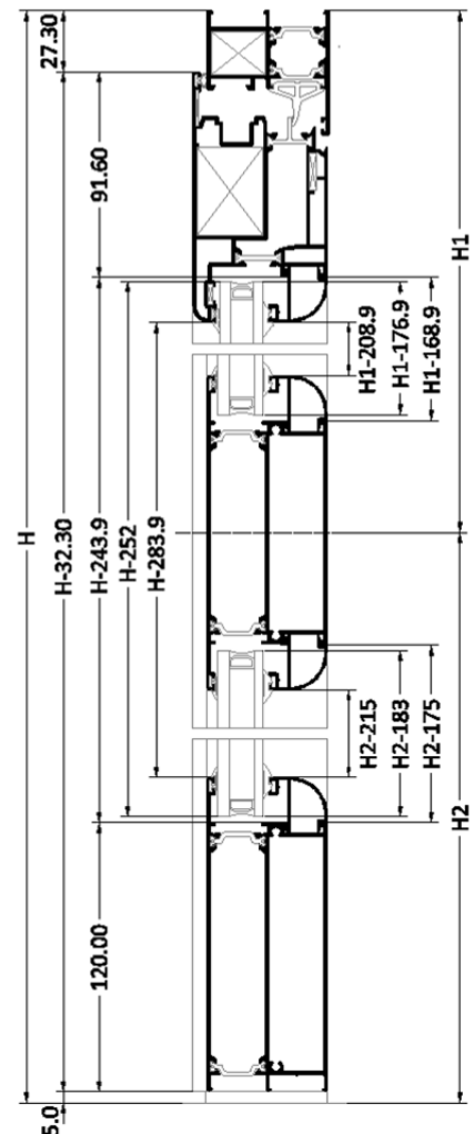
SECCION VERTICAL B-B'
