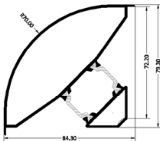
ESQUINERO MARCOS 54 Y 59 MM CAN/16
