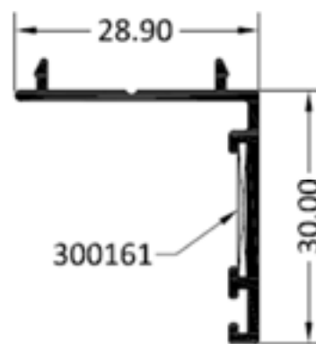
SOLAPE CLIPADO DE 30 MM
