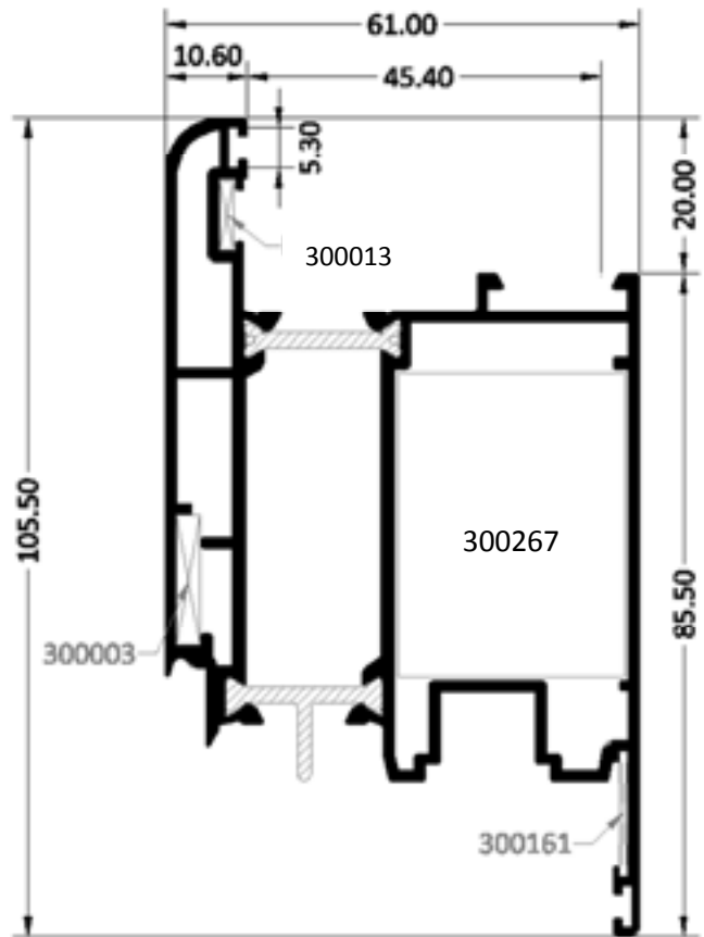
HOJA PUERTA AP. INT. CAN/16
