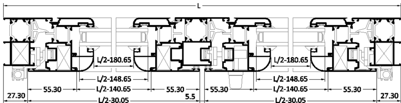
SECCION HORIZONTAL B-B'
