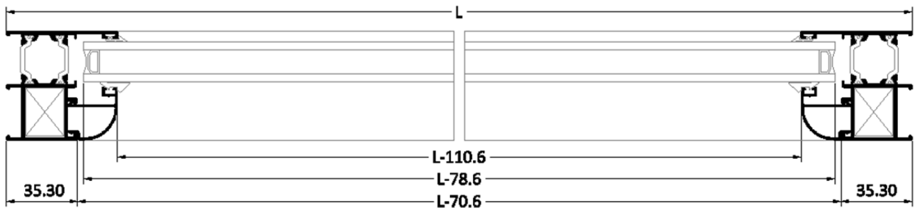
SECCION HORIZONTAL B-B'
