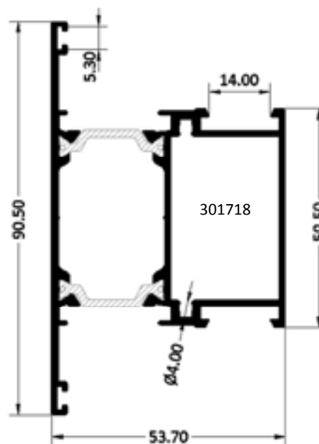
TRAVESAÑO PUERTA 67 MM CAN/16
