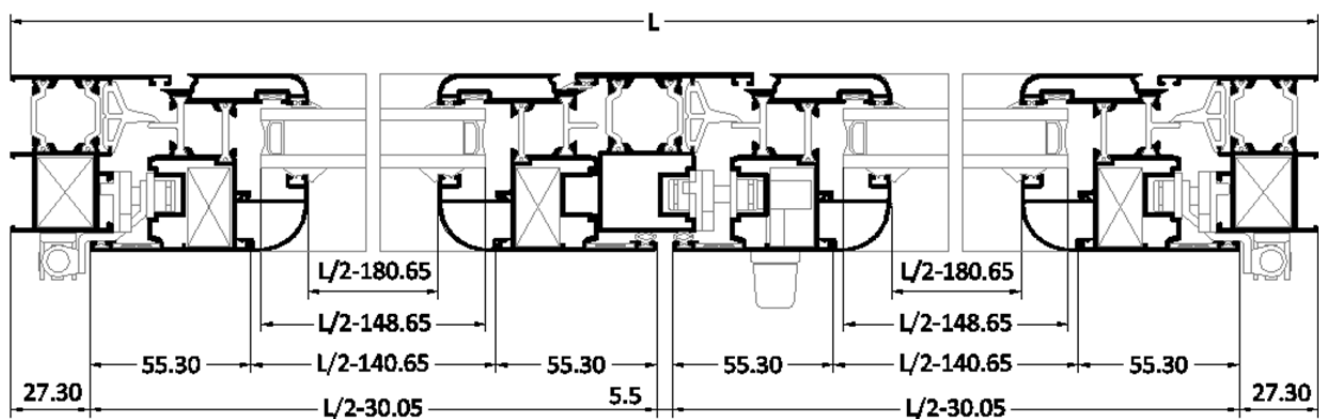
SECCION HORIZONTAL A-A'
