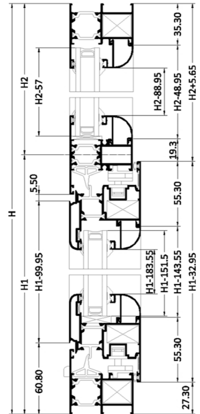
SECCION VERTICAL B-B'
