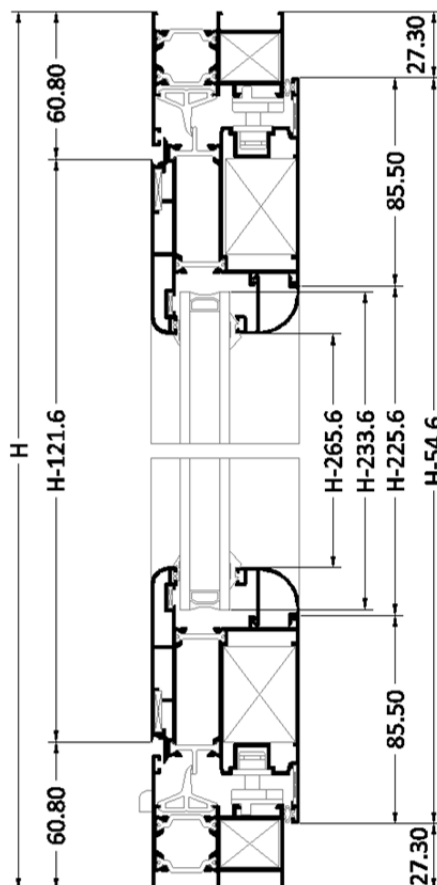
SECCION VERTICAL B-B'
