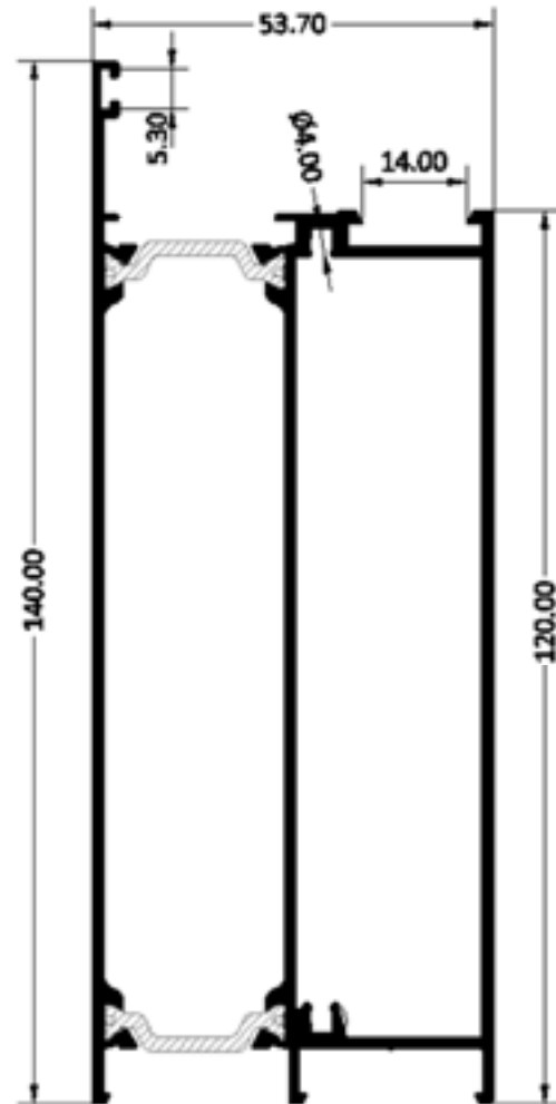
ZÓCALO 140 MM CAN/16
