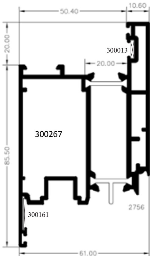
HOJA PUERTA RECTA AP. INT. CAN/16
