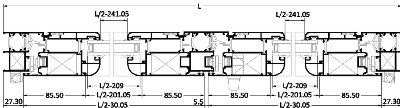
SECCION HORIZONTAL A-A'
